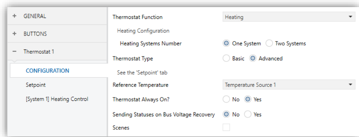
Figura 33 Thermostat.
